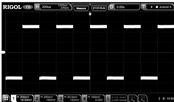
Осциллограмма до усреднения
